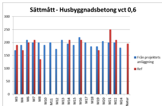
Figur 11 Sättningsmått för testade betonger
