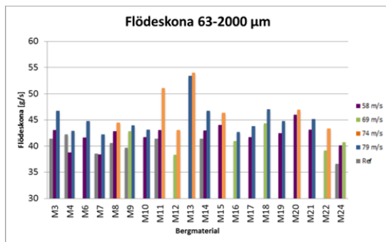
Figur 4 Flödeskonans beroende av VSI hastighet
